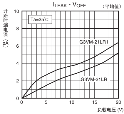
●开路时漏电流—负载电压 G3VM-21LR/21LR1
