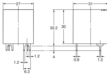
基板安装状态(参考)
