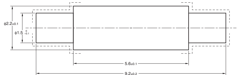
促动器设计参考图
