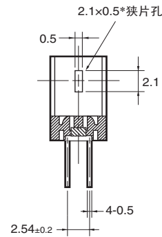
断面AA *输入侧、输出侧尺寸相同
