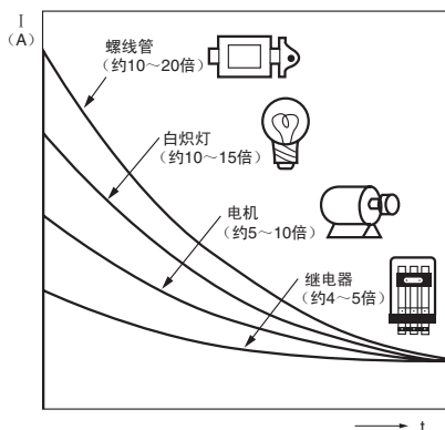
负载的种类和浪涌电流
