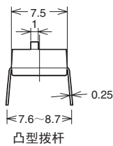
单极侧面图
