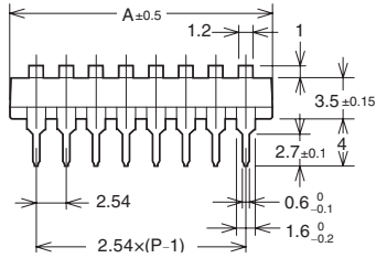
凸型拨杆
