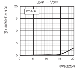
개로시 누설전류-부하전압
