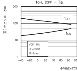
동작, 복귀시간-주위온도
