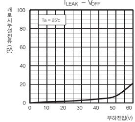
개로시 누설전류-부하전압
