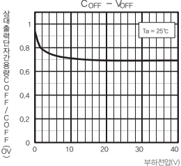
상대출력단자간용량-부하전압
