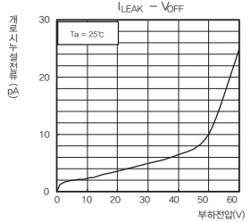
개로시 누설전류-부하전압
