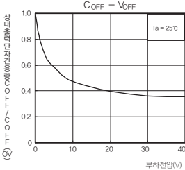
상대출력단자간용량-부하전압
