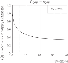
상대출력단자용량-부하전압
