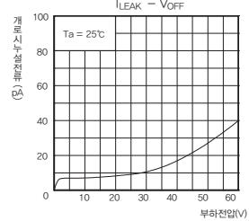
개로서 누설전류-부하전압
