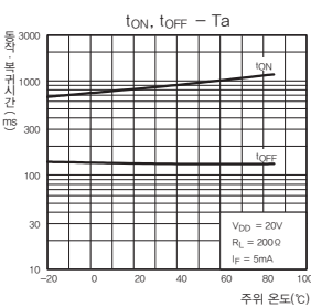
동작, 복귀시간-주위온도
