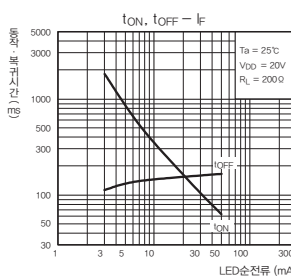
동작, 복귀시간-LED순전류
