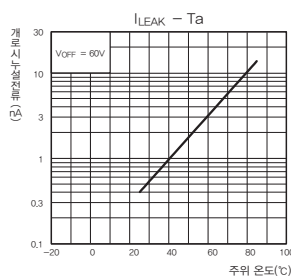
개로시 누설전류-주위온도
