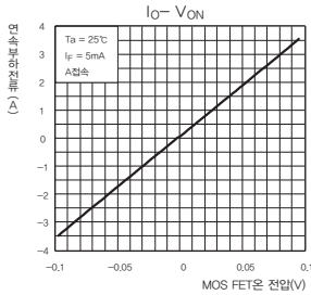
연속부하전류-MOS FET ON전압
