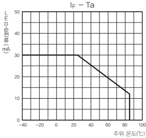
LED순전류-주위온도
