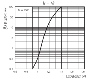
LED순전류-LED순전압
