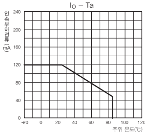
연속부하전류-주위온도
