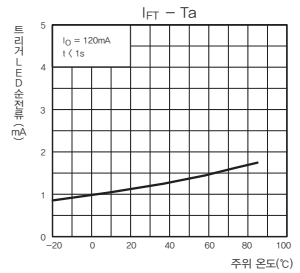
트리거LED순전류-주위온도
