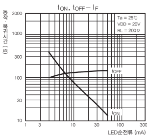
동작, 복귀시간-LED순전류
