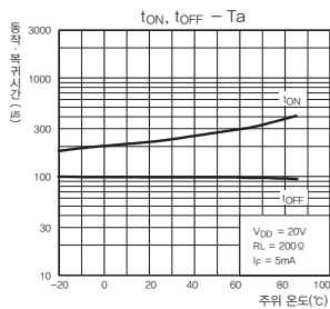
동작, 복귀시간-주위온도
