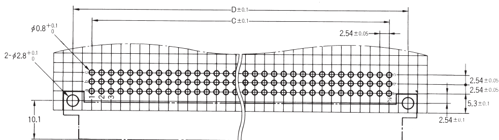
プリント基板加工寸法 (BOTTOM VIEW)
