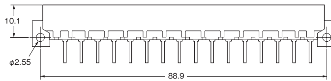
プリント基板加工寸法 (BOTTOM VIEW)
