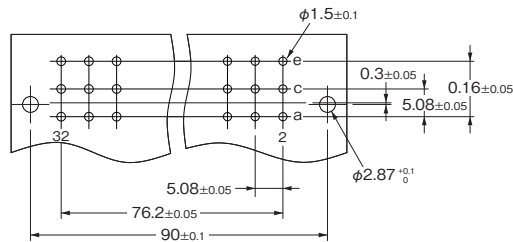
プリント基板加工寸法 (BOTTOM VIEW)
