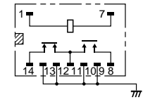
端子配置/内部接続図 (BOTTOM VIEW)
