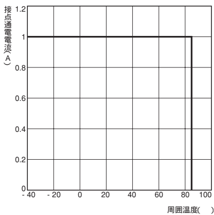
周囲温度と接点通電電流
