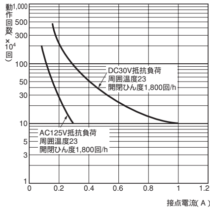
耐久性曲線
