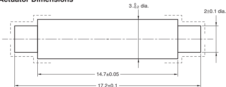
Actuator Dimensions
