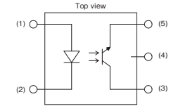
内部回路
